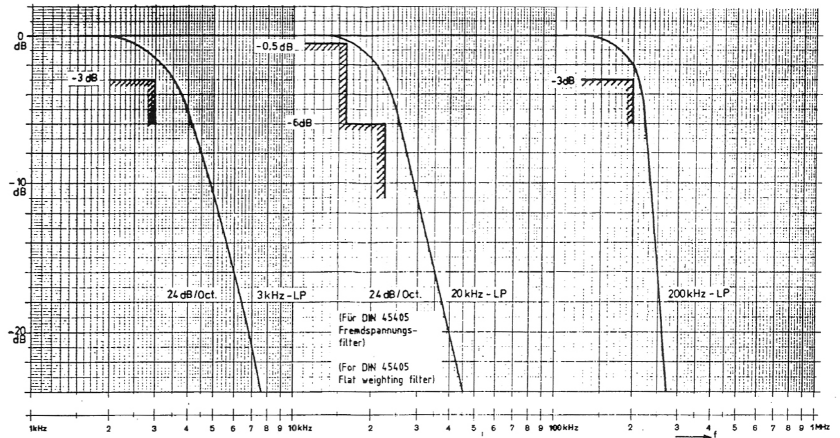
Bild 2-7 FAM Tiefpaß-Filterkurven Fig. 2-7 FAM Low pass filter characteristics
