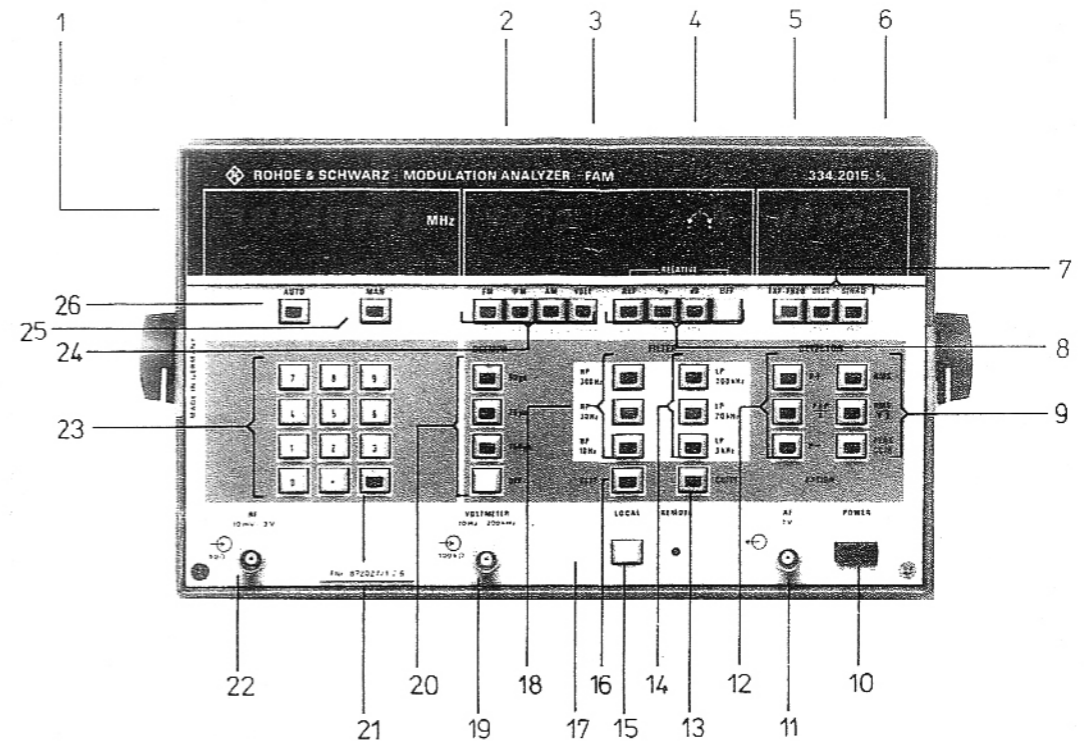
Bild 2-5 Frontansicht Fig. 2-5 Front view
