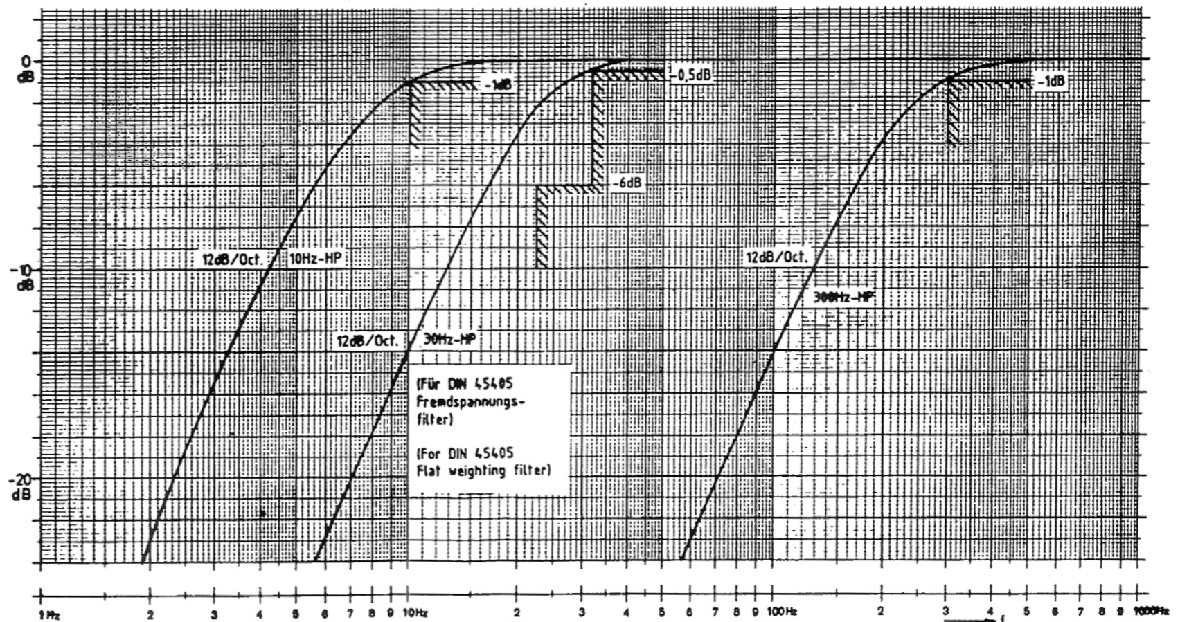
Bild 2-8 FAM Hochpaß-Filterkurven Fig. 2-8 FAM High pass filter characteristics
