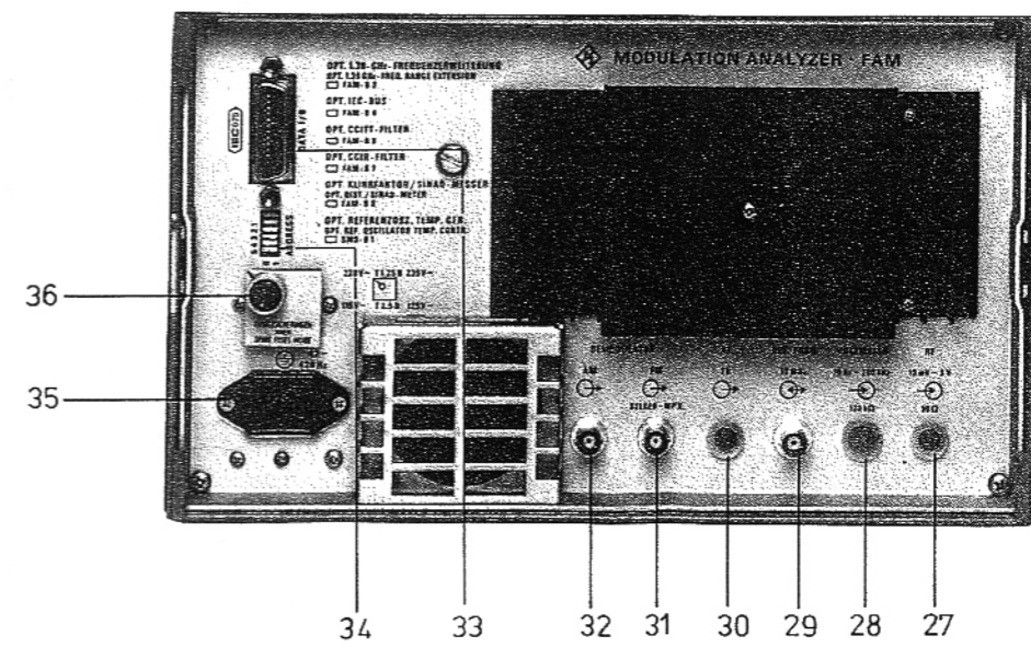
Bild 2-6 Rückansicht Fig. 2-6 Rear view
